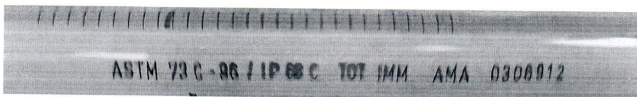
Рисунок 1.2 – Фотография маркировки термометра ртутного стеклянного ASTM 73 C № 0306912
