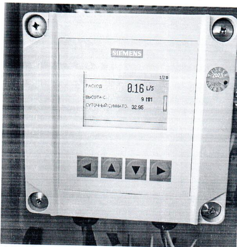
Рисунок 1.1 – Фотография общего вида уровнемера ультразвукового SITRANS LUT 440 № PBD/L6270481 входящего в состав узла учета
