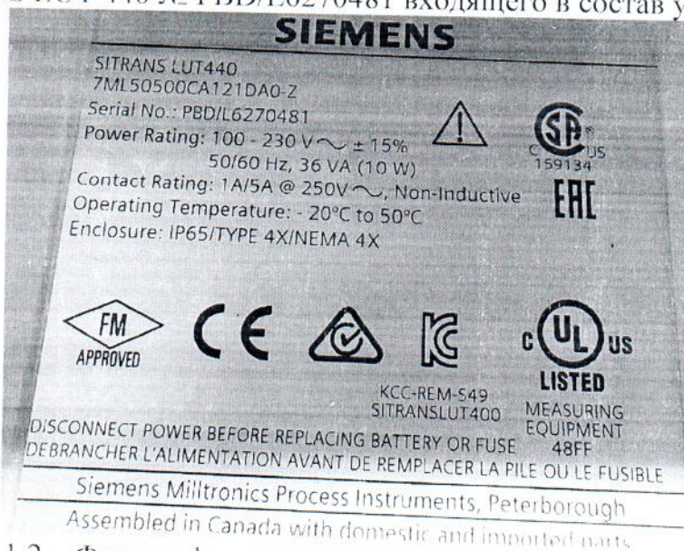
Рисунок 1.2 – Фотография маркировки уровнемера ультразвукового SITRANS LUT 440 № PBD/L6270481 входящего в состав узла учета
