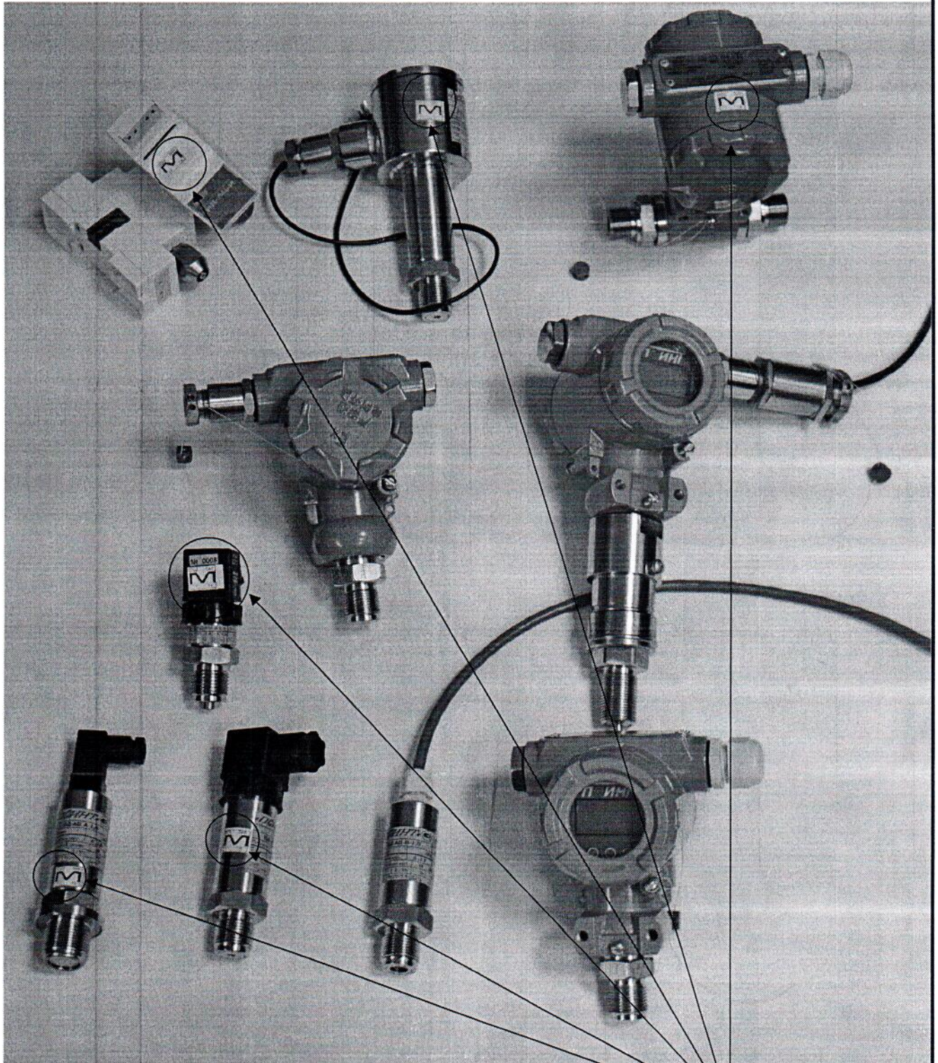
Рисунок А1 - Внешний вид датчиков давления ИД и место нанесения знака поверки в виде клейма-наклейки
