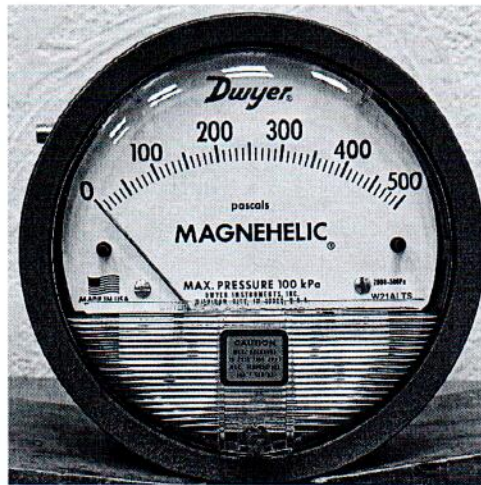
Рисунок 1.1 – Фотография общего вида манометра дифференциального показывающего Magnehelic 2000-500PA № 1302723СК-36
