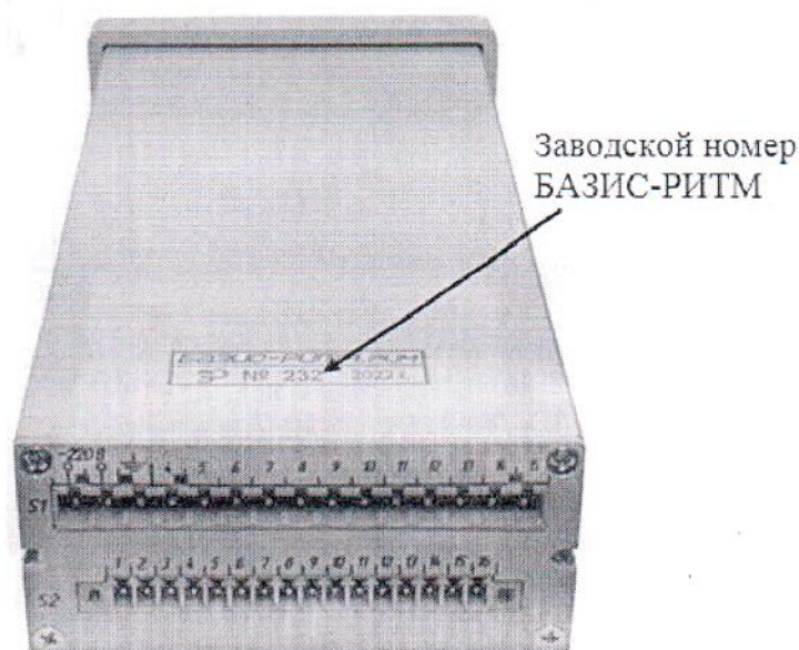
Рисунок 2 – Расположение заводского номера на корпусе БАЗИС-РИТМ
