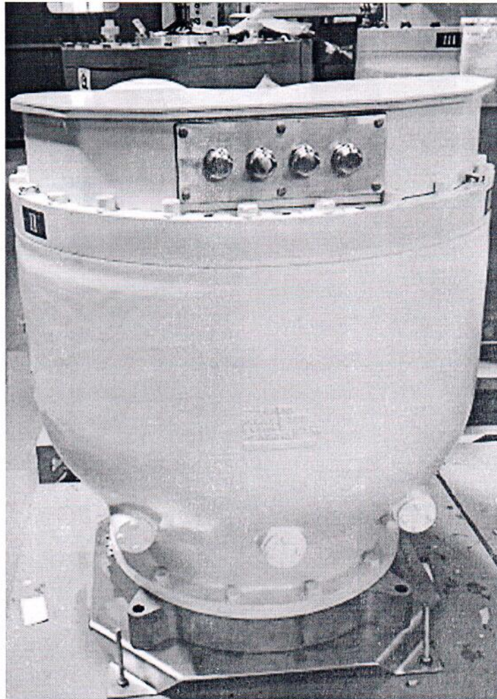
Рисунок 1.1 – Фотографии общего вида трансформатора напряжения SU145/S92 № 1VT566
