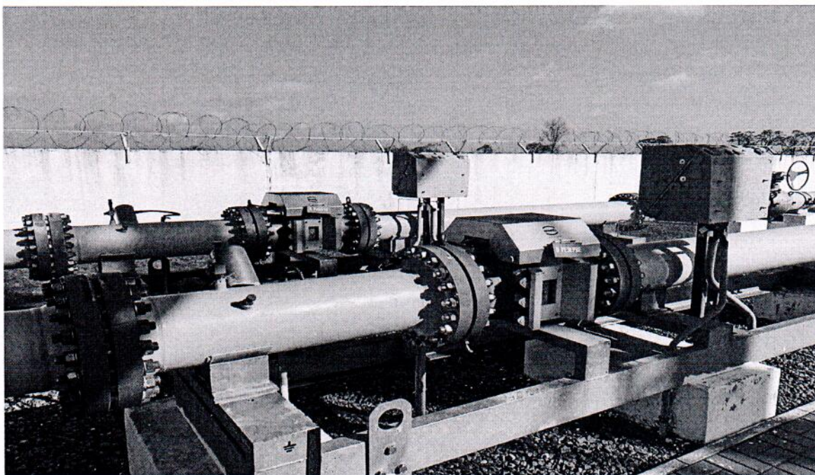
Рисунок 1.1 – Фотографии общего вида ИС УУГ
