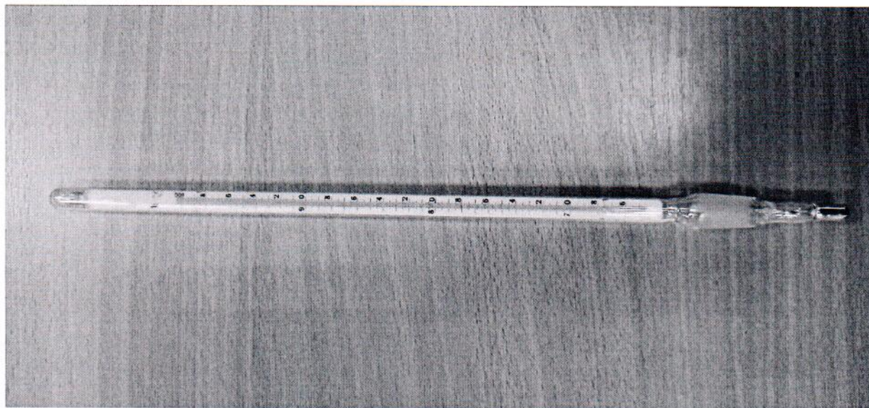
Рисунок 1.1 – Фотография общего вида термометра лабораторного стеклянного с взаимозаменяемыми конусами № 3, заводской № 12
