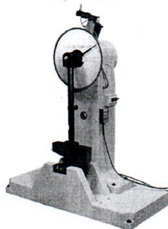
Рисунок 4 – Общий вид копров маятниковых ГОСТ серии МИК модификации МИК-150 (300; 450; 750; 900). 2-1.1.У
