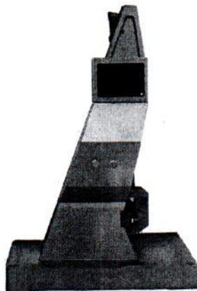
Рисунок 5 – Общий вид копров маятниковых ГОСТ серии МИК модификации МИК-150 (300; 450; 750; 900). 2-2.2.V
