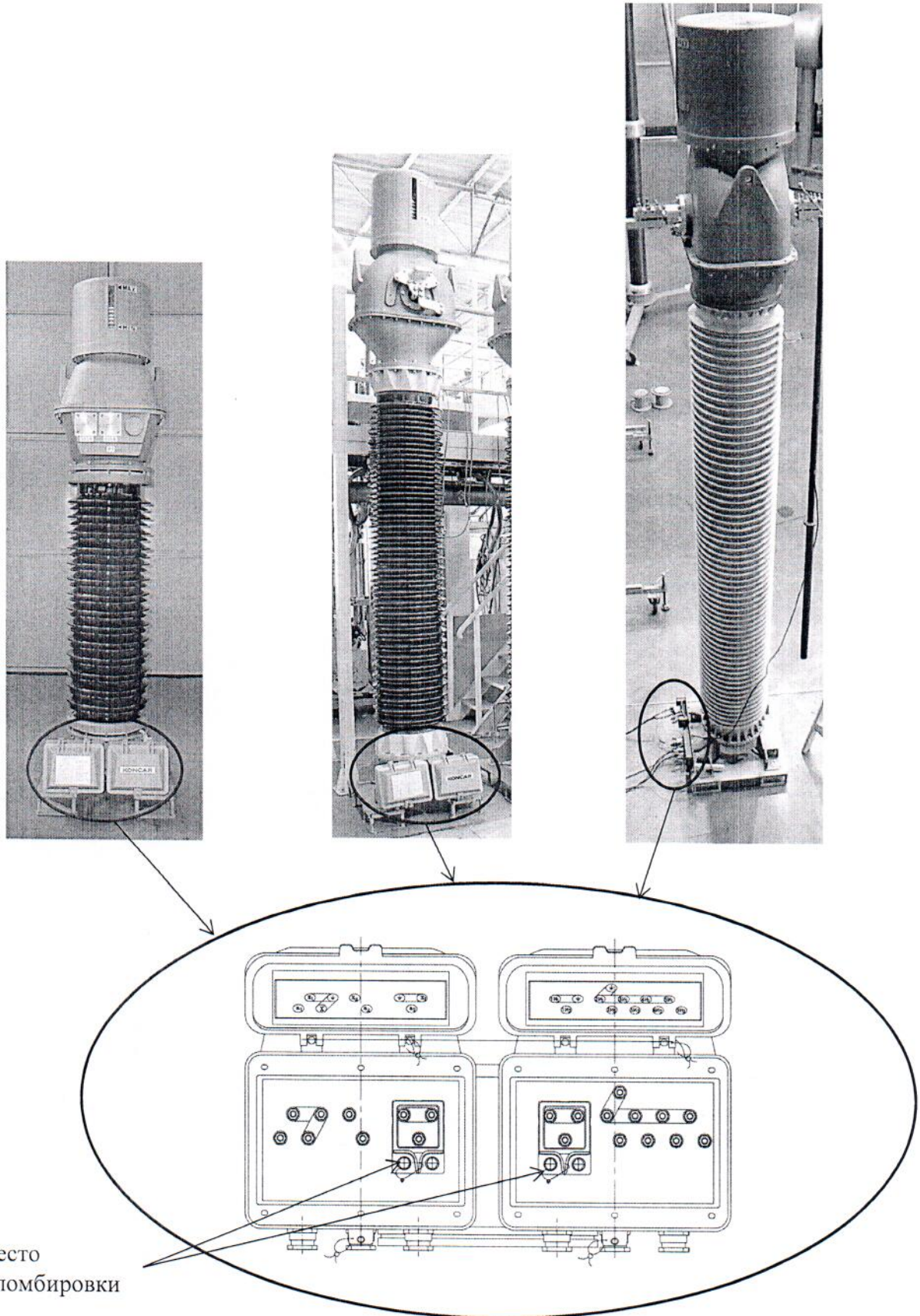
Рисунок 2 Схема пломбировки трансформаторов VAU-123, VAU -245, VAU -362.
