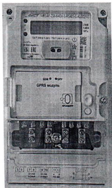
Рисунок 1.3 – Фотография общего вида счётчика в исполнении корпуса W3
