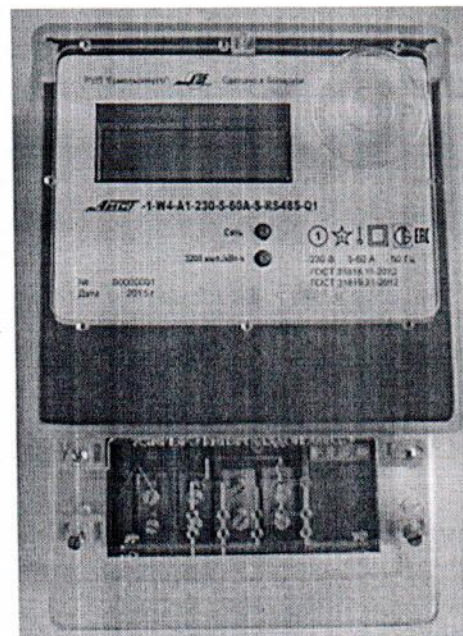
Рисунок 1.4 – Фотография общего вида счётчика в исполнении корпуса W4
