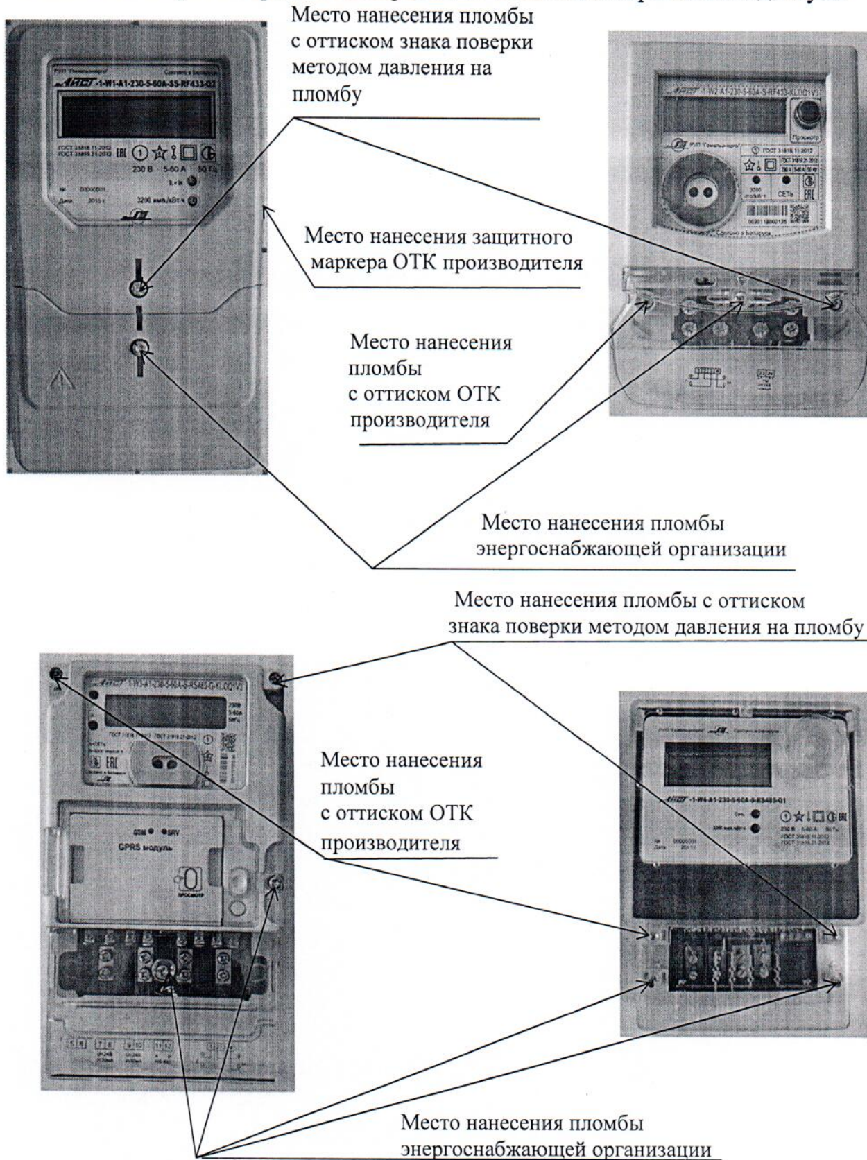
Рисунок 3.1 - Схема пломбировки счётчиков от несанкционированного доступа
