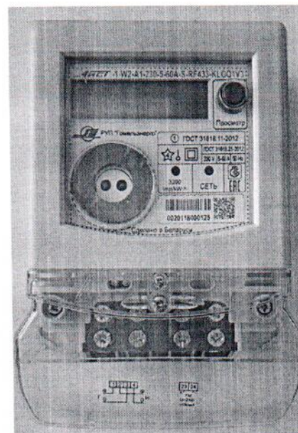
Рисунок 1.2 – Фотография общего вида счётчика в исполнении корпуса W2
