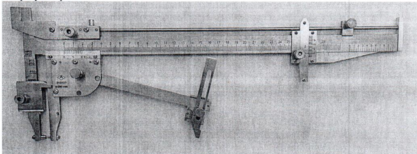
Рисунок 1 – Общий вид штангенциркулей путевых ПШВ-01
