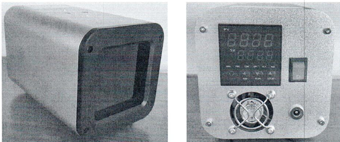
Рисунок 1.1 – Общий вид абсолютно черного тела Sunell SN-TH01 № S125822009014720003
