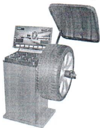
Рисунок 2 - Общий вид станков балансировочных LC131
