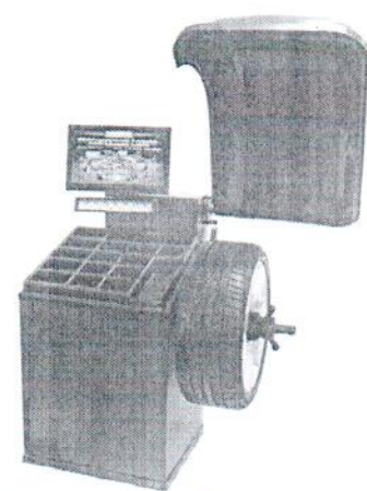
Рисунок 4 - Общий вид станков балансировочных LC432
