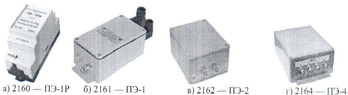
Рисунок 4 – Пневмоэлектрические преобразователи ПЭ.
