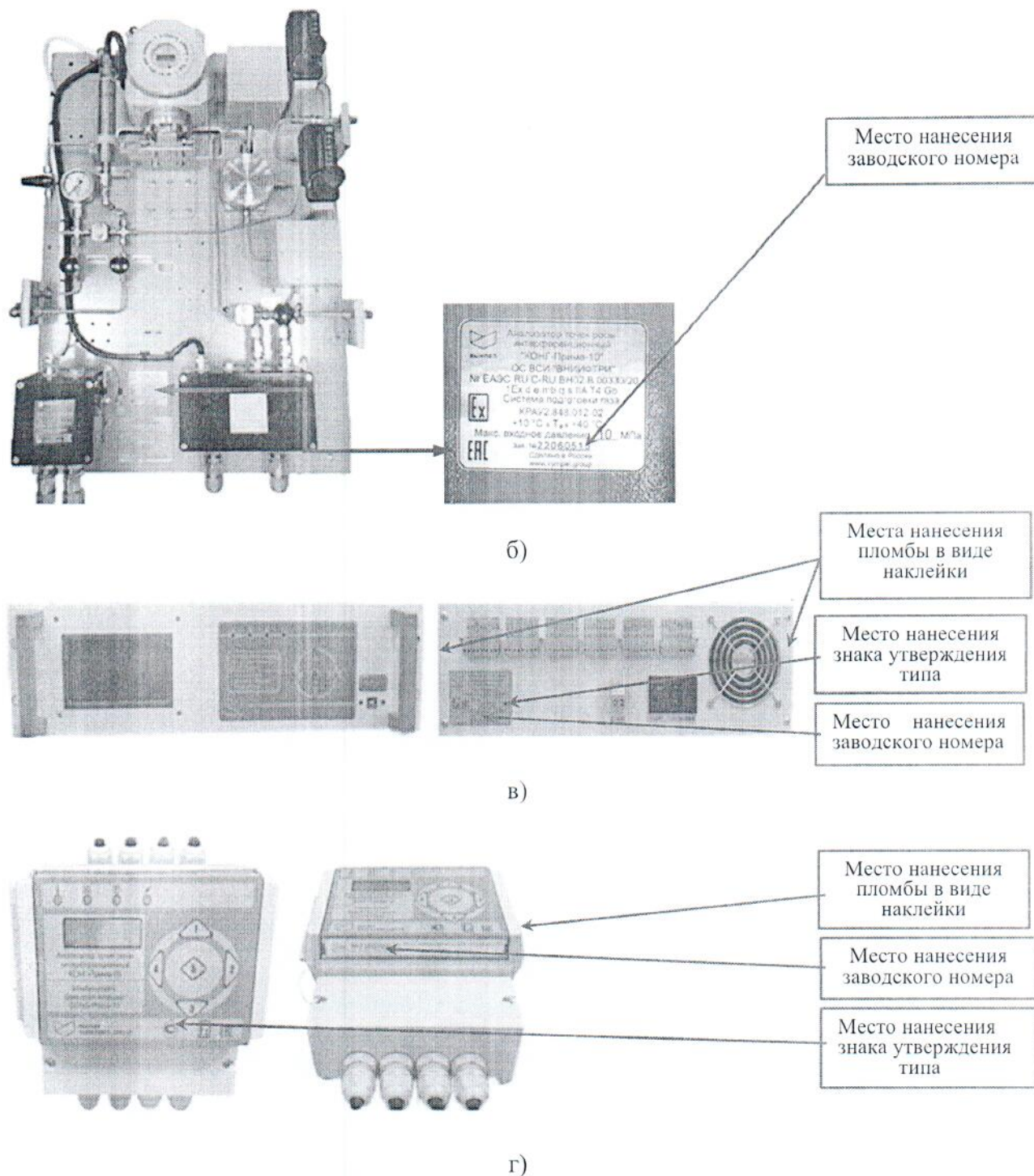
Рисунок 1 - Общий вид средства измерений с указанием мест пломбировки от несанкционированного доступа, нанесения заводского номера и знака утверждения типа
