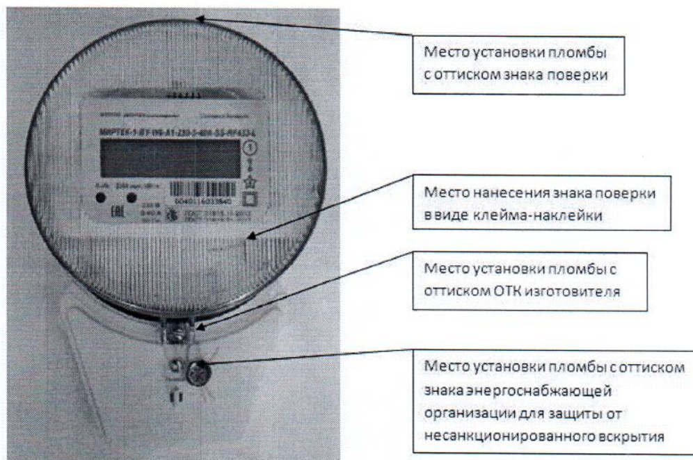
Рисунок Б.6 – Места установки пломб и нанесения знака поверки для счетчиков в корпусе W6
