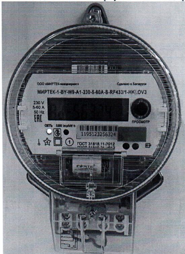
Рисунок А.12 - Внешний вид счетчика в корпусе W9 с модификацией ЖКИ № 1
