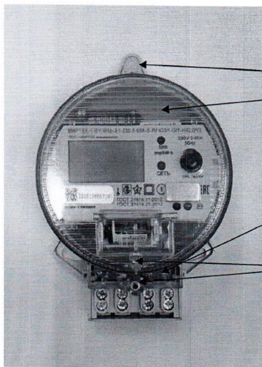
Рисунок Б.7 – Места установки пломб и нанесения знака поверки для счетчиков в корпусе W6b
