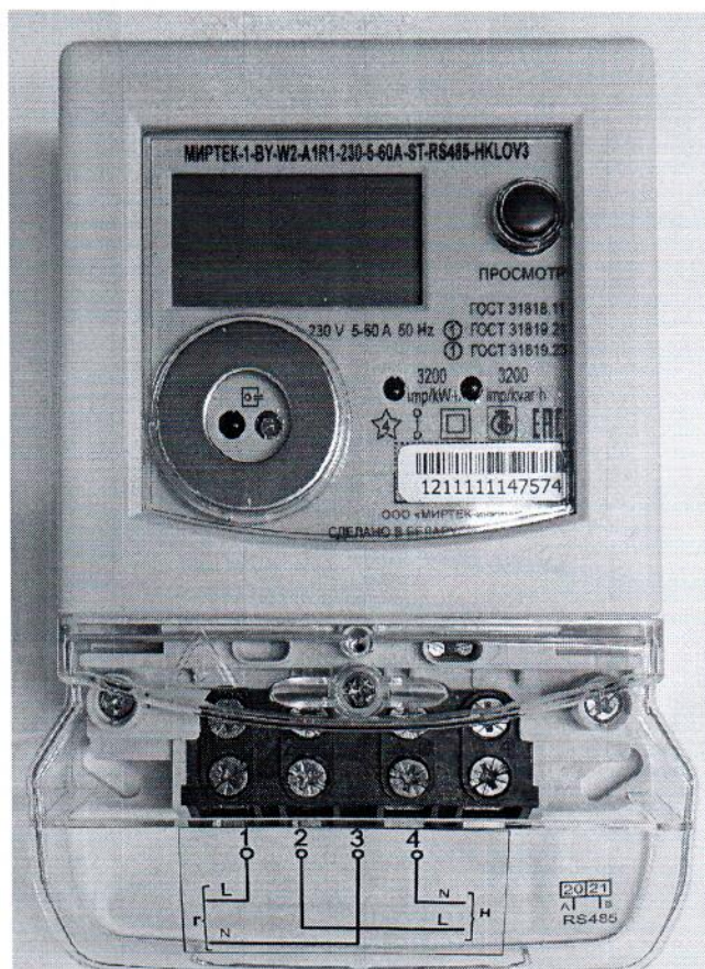
Рисунок А.3 – Внешний вид счетчика в корпусе W2 с модификацией ЖКИ № 2
