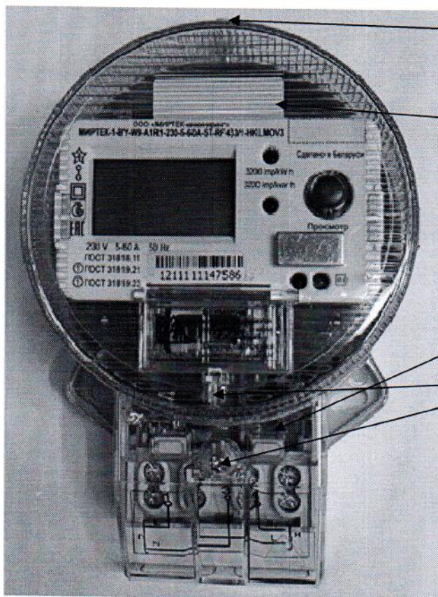
Рисунок Б.8 – Места установки пломб и нанесения знака поверки для счетчиков в корпусе W9
