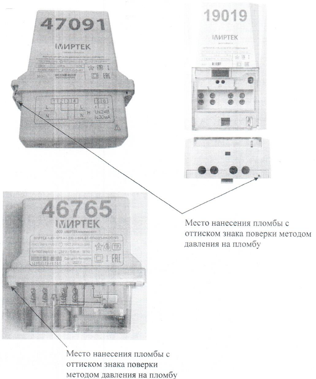
Рисунок 3.1 - Схема (рисунок) с указанием места для нанесения знака поверки методом давления на пломбу и схема пломбировки средств измерений от несанкционированного доступа для счетчиков «МИРТЕК-1-ВУ-СП»
