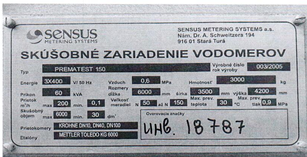
Рисунок 1.2 – Фотография маркировки установки поверочной расходомерной Prematest 150 № 003/2005
