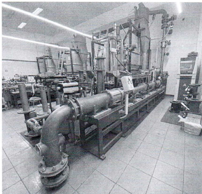
Рисунок 1.1 – Фотография общего вида установки поверочной расходомерной Prematest 150 № 003/2005
