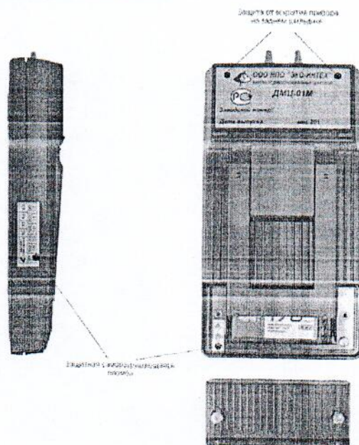
Рис. 2. Места наклеивания пломбы и перфорации на заднем шильдике для защиты от вскрытия.
