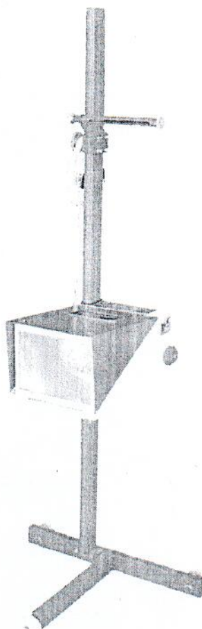
Общий вид измерителей параметров света фар автотранспортных средств ИПФ-01
