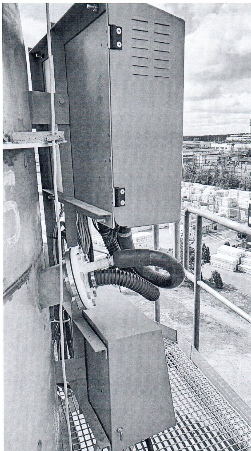
Рисунок 1.5 – Фотография общего вида подсистемы измерения концентрации твердых частиц в дымовых газах АСКВ с анализатором пыли DUSHUNTER FWE200DH
