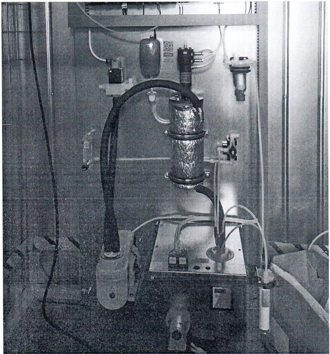
Рисунок 1.2 – Фотография общего вида подсистемы отбора и транспортировки пробы
