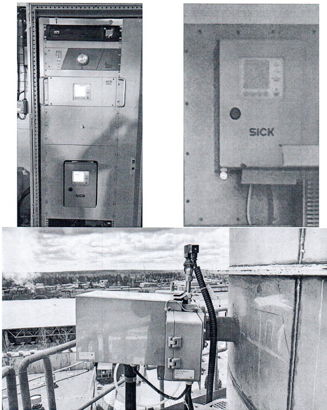
Рисунок 1.3 – Фотографии общего вида подсистемы измерения концентраций газов АСКВ с газоанализатором GSM 810 с модулями и анализатором кислорода ТДК-3М
