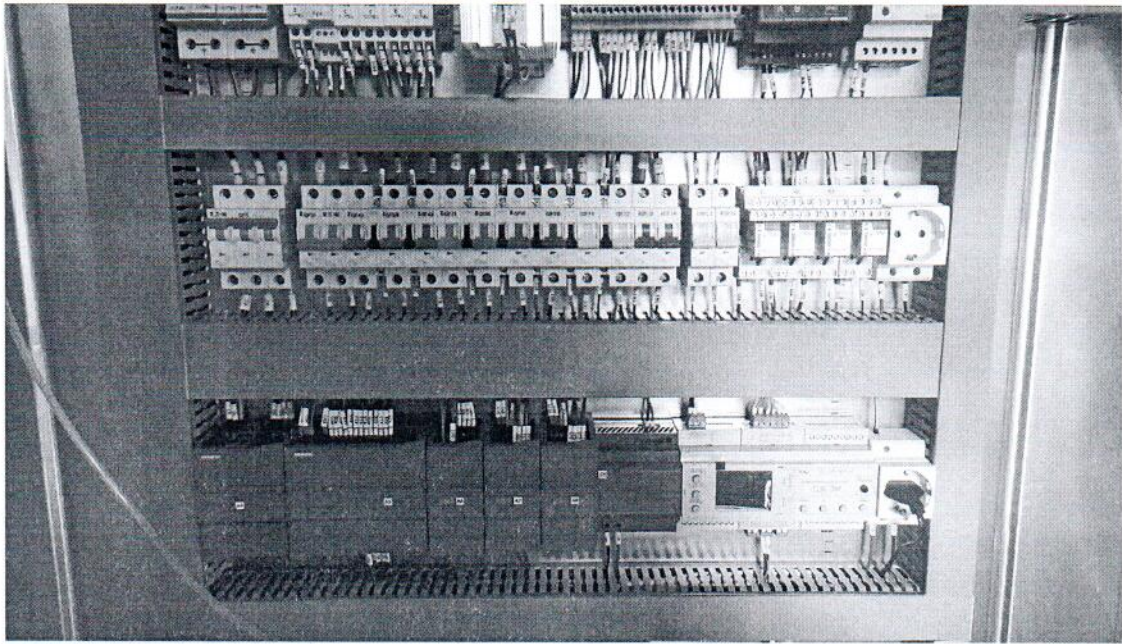
Рисунок 1.6 – Фотография общего вида подсистемы сбора и передачи данных АСКВ
