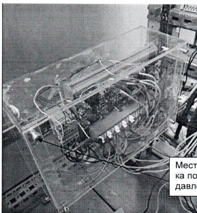
Рисунок 3.4 – Места пломбировки модуля нормализации частотных сигналов TVA 8-6
