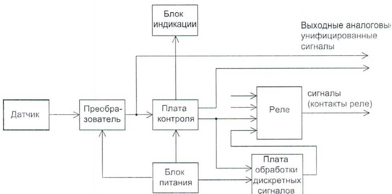
Рисунок 2 - Структурная схема
