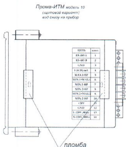
Рис.1. Схема пломбировки измерителя ПРОМА-ИТМ
