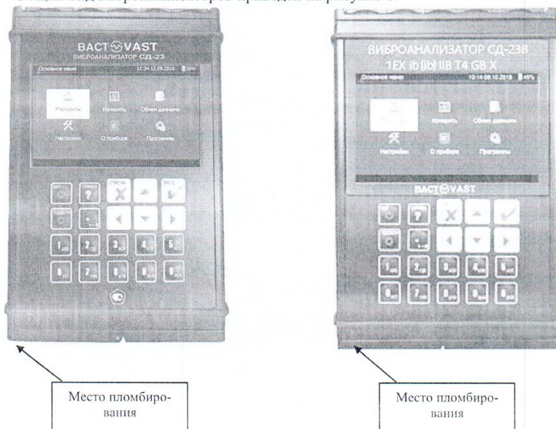
Рисунок 1 – Общий вид и место пломбирования виброанализаторов СД-23 и СД-23В
