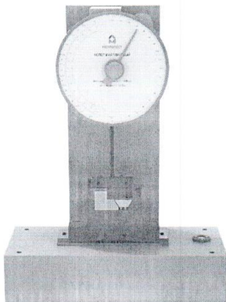
Рисунок 3 – Общий вид копра маятникового KM-5 (25/50)-P-Ш
