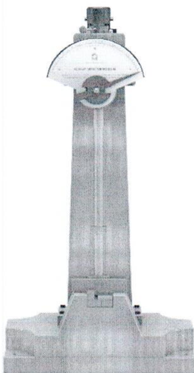
Рисунок 5 – Общий вид копра маятникового KM-150(300/450)-P-Ш
