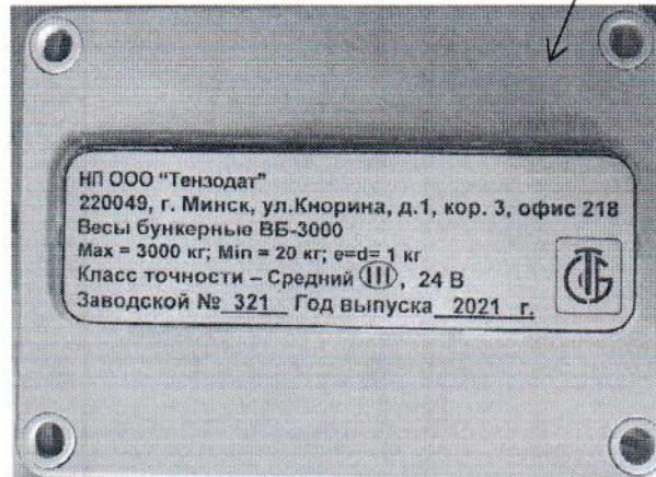
Рисунок 2.1 - Фотография с указанием места нанесения знака поверки (наклейки) на преобразователь тензометрический ТПН-1
