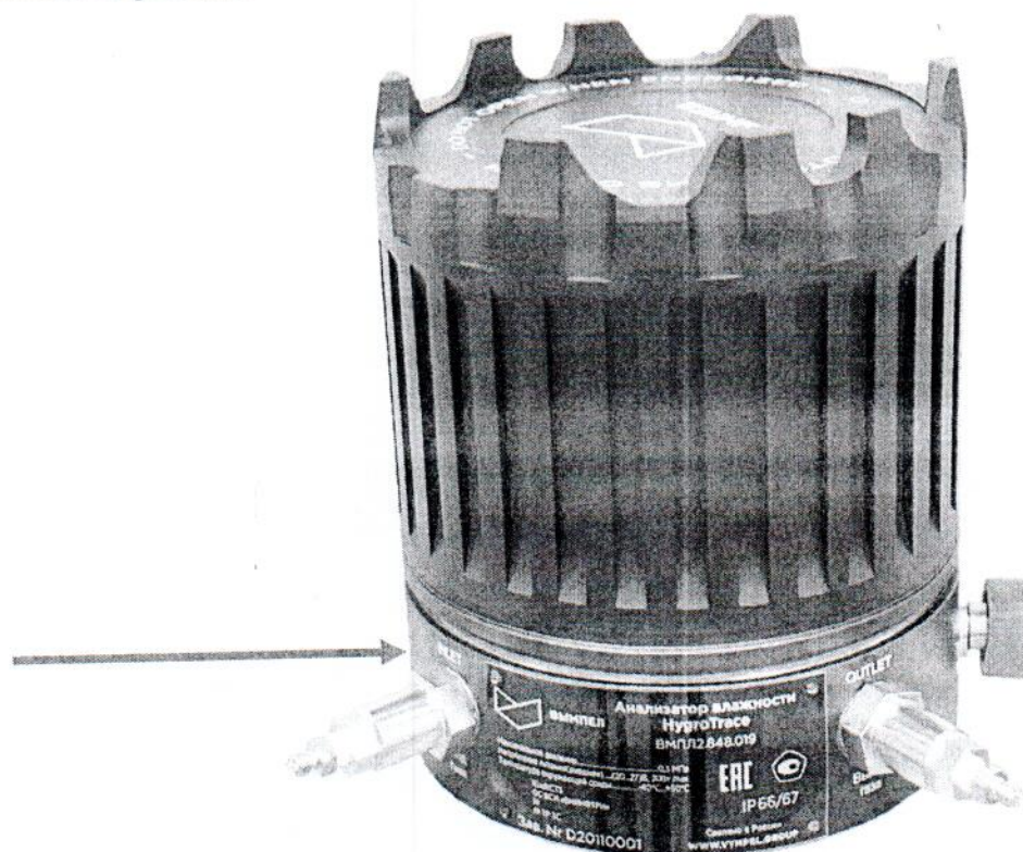
Рисунок 1 – Общий вид анализатора влажности HygroTrace, место нанесения знака поверки
