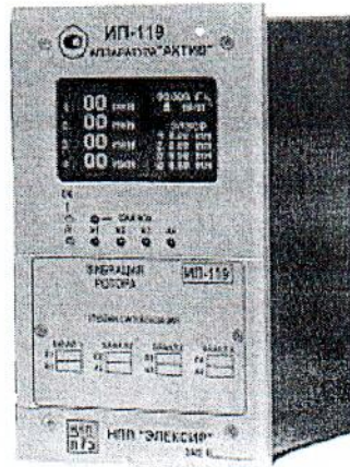
Блок ИП- 119
