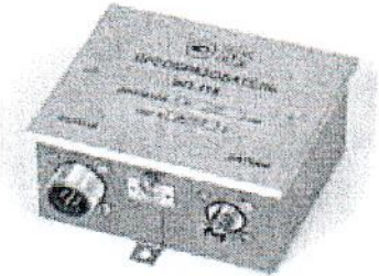
Преобразователь ИП-116
