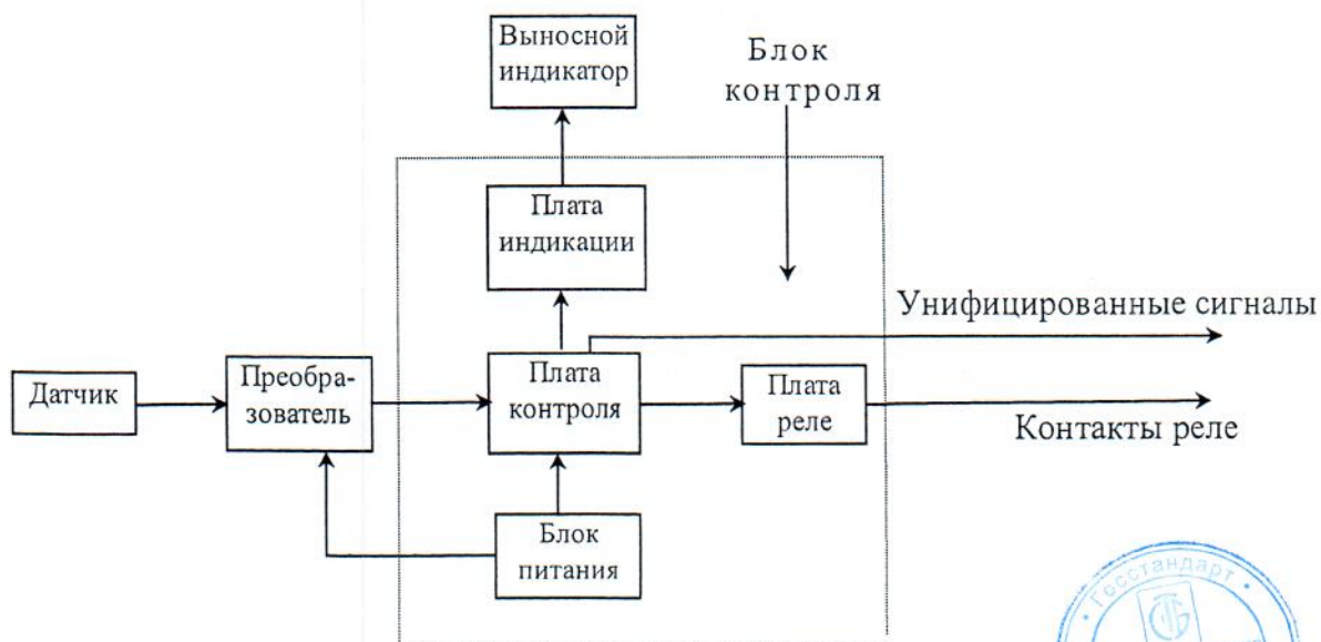
Рисунок 2 - Структурная схема измерительного канала аппаратуры «АКТИВ»
