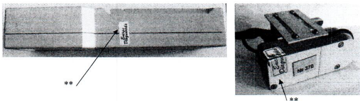
Рисунок 2 – Схема пломбирования от несанкционированного доступа измерителя концентрации напряжений ИКН (на примере ИКН-3М-12) и измерительного датчика.
