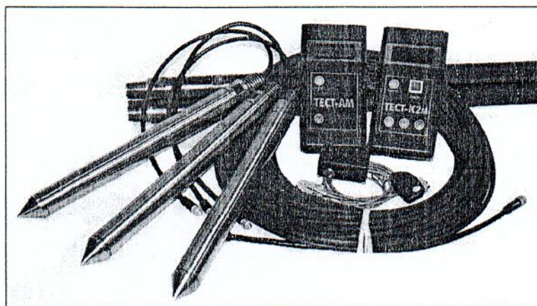
Рисунок 1 - Общий вид аппаратуры ТЕСТ
