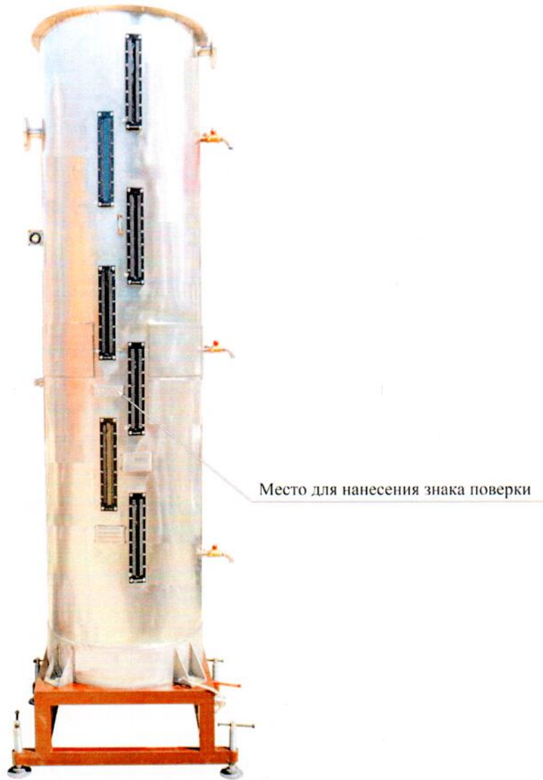
Рисунок 2 – Указание места для нанесения знака поверки мерника технического 1-го класса М1кл-750 № 12
