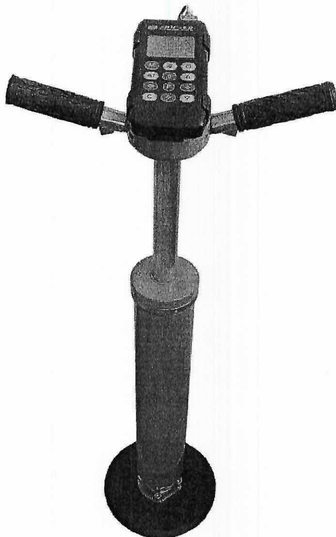
Рисунок 3 - Общий вид измерителя динамического модуля упругости грунтов ДПГ (модификация ДПГ-1.1)
