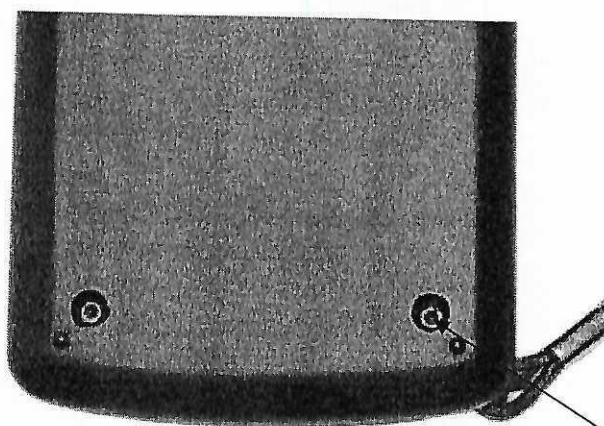
Рисунок 2 - Место пломбирования и клеймения измерителей модификаций ДПГ-1.2
