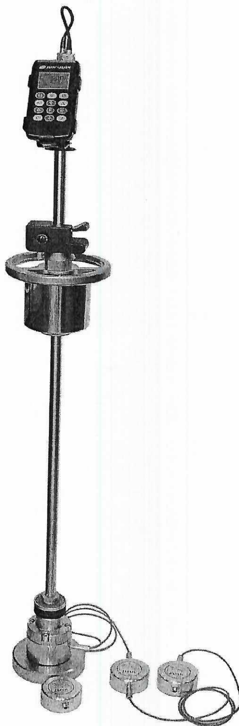
Рисунок 5 - Общий вид измерителя динамического модуля упругости грунтов ДПГ (модификация ДПГ-ДДК)
