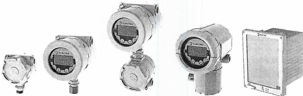
Рисунок 2 – Конструктивные исполнения модулей электронного преобразователя расходомера Примечание – цветовая гамма может отличаться в зависимости от типа покрытия и требований заказчиков
