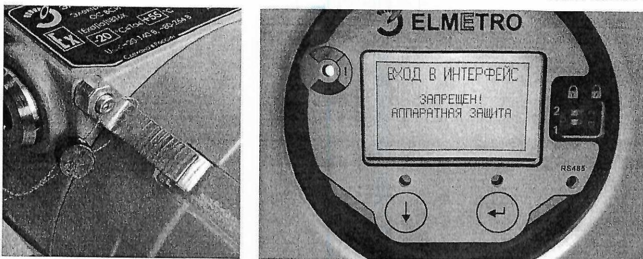
Рисунок 3 – Место пломбирования расходомера и сообщение на дисплее при запрещающем положении микропереключателей
