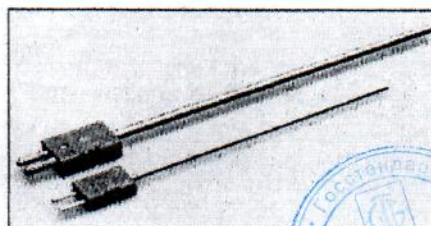
Рисунок 2 - Общий вид ДТТ с кабельными выводами модификации ХХ4
