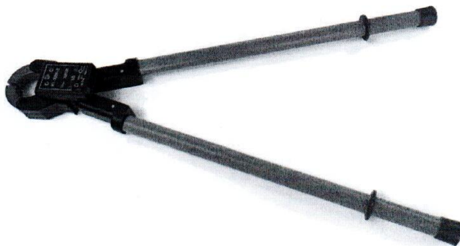
Рисунок 7 – Общий вид клещей токоизмерительных КТ-1000-В (с ручками)
