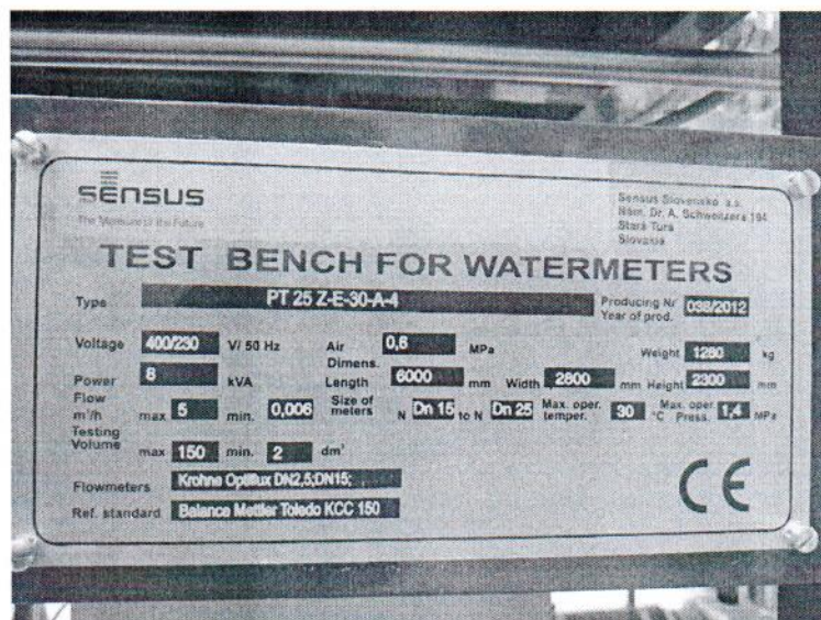
Рисунок 2 – Фотография маркировки установки
