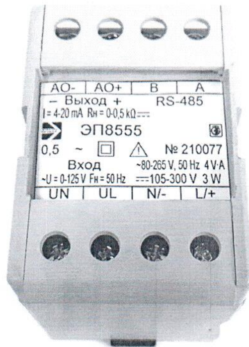
Рисунок 1.3 – ЭП8555 в корпусе с габаритными размерами 55x81x71 мм
