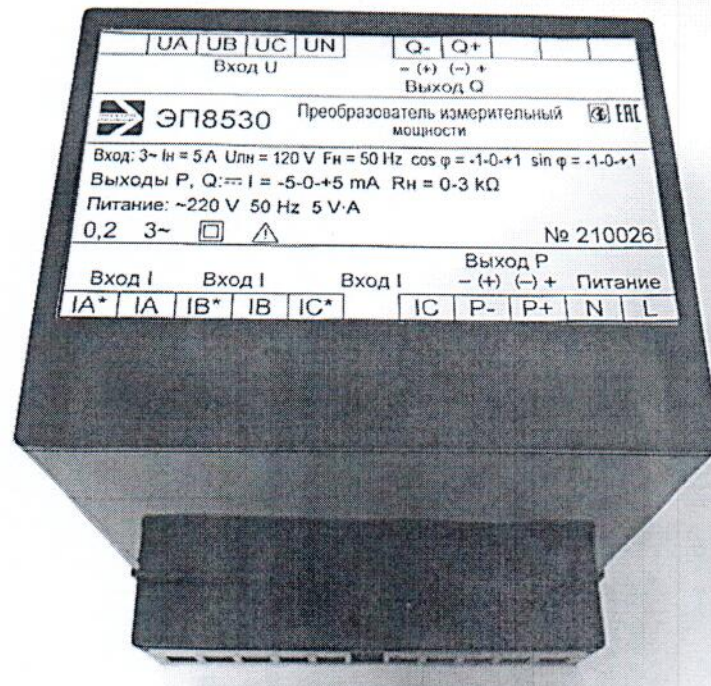
Рисунок 1.4 – ЭП8530 в корпусе с габаритными размерами 125x90x125 мм
