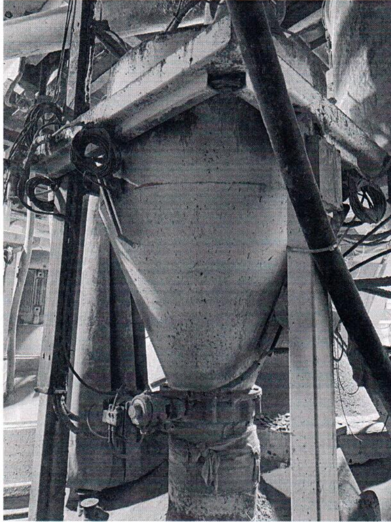
Рисунок 1.1 – Внешний вид дозатора весового дискретного действия цемента ДВДДц-1000 №11702658_4
