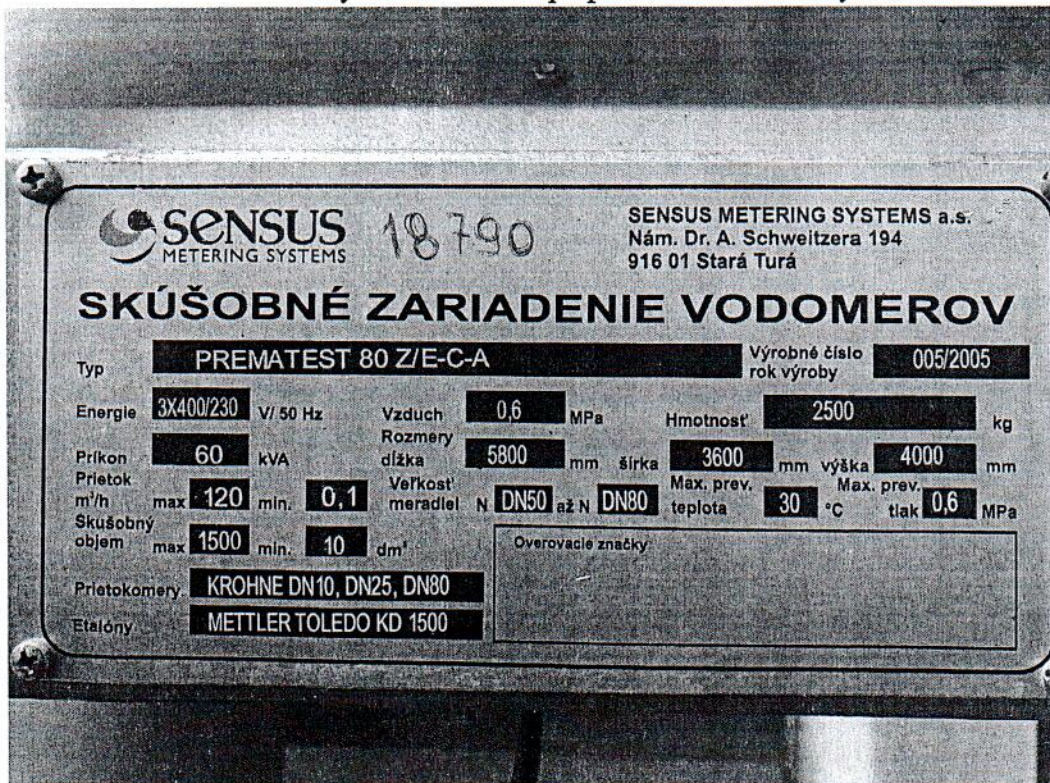
Рисунок 2 – Фотография маркировки установки
