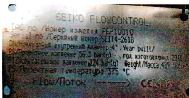
Рисунок А.3 – Маркировка клинового расходомера SEIKO № FE-10010
