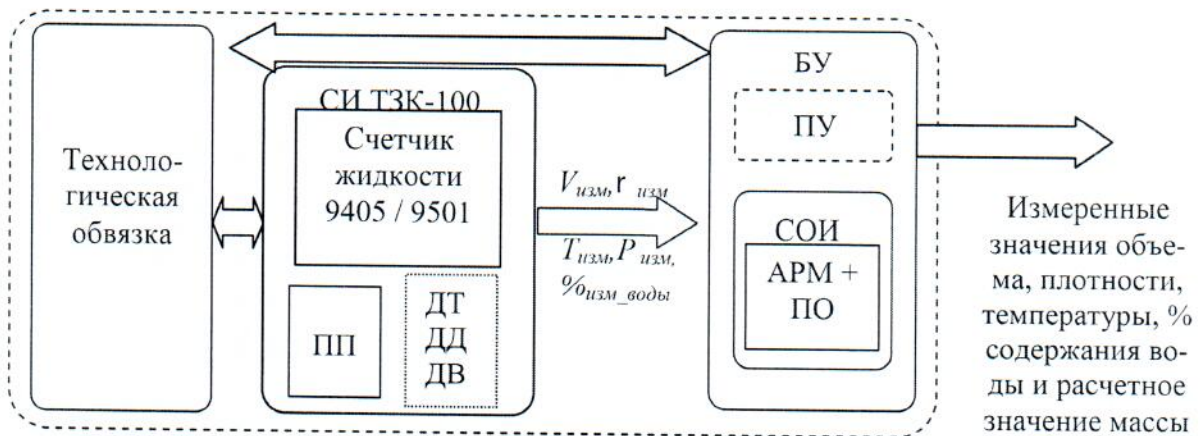
Рисунок 4 – СИ ТЗК - 100 ОПXXXX, ТЗК - 100 ОПXXXX-В
