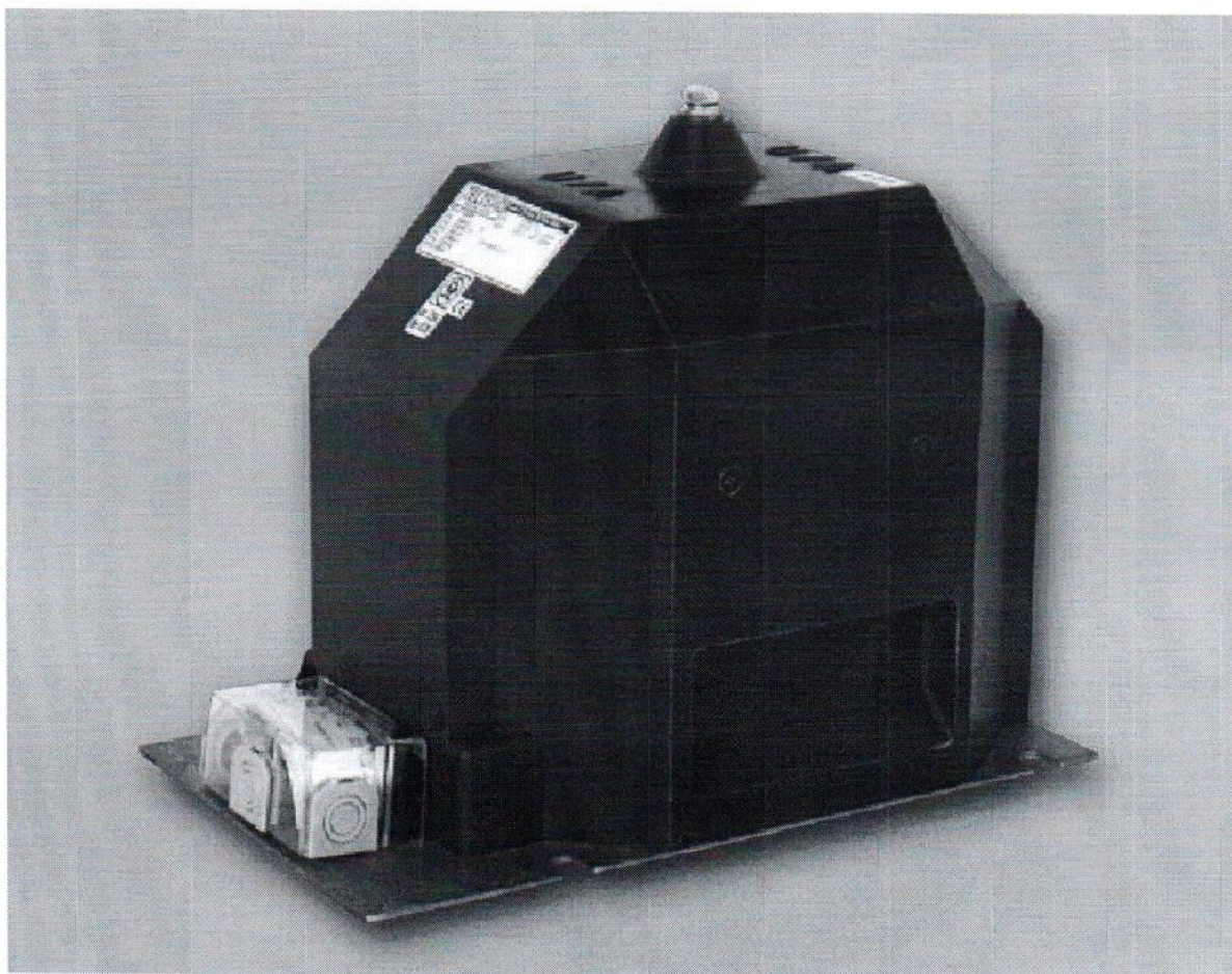
Рисунок 1 – Внешний вид трансформатора напряжения измерительного 4MR (EGS, EGG)
