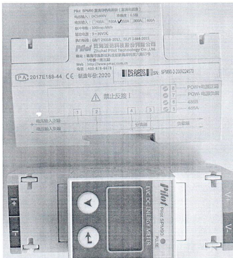
Рисунок 1.1 – Внешний вид счетчика SPM90 зав. № SPM90-2-2009224570
