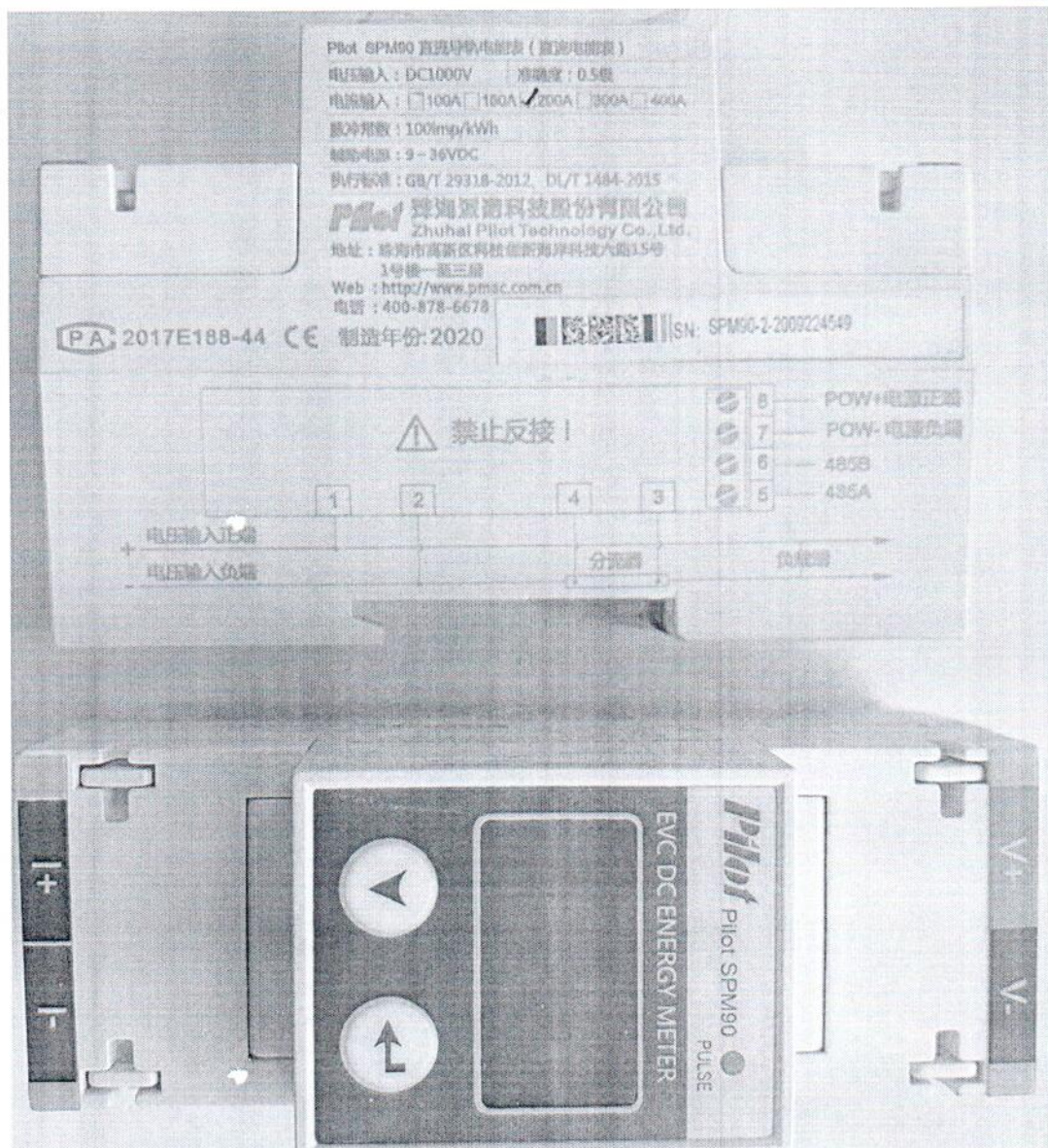
Рисунок 1.1 – Внешний вид счетчика SPM90 зав. № SPM90-2-2009224549
