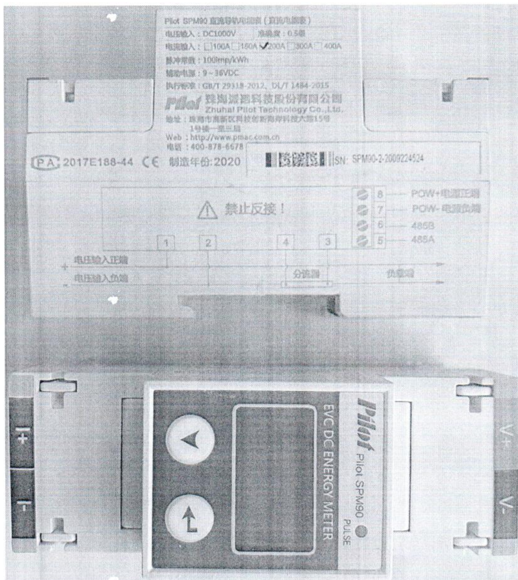
Рисунок 1.1 – Внешний вид счетчика SPM90 зав. № SPM90-2-2009224524
