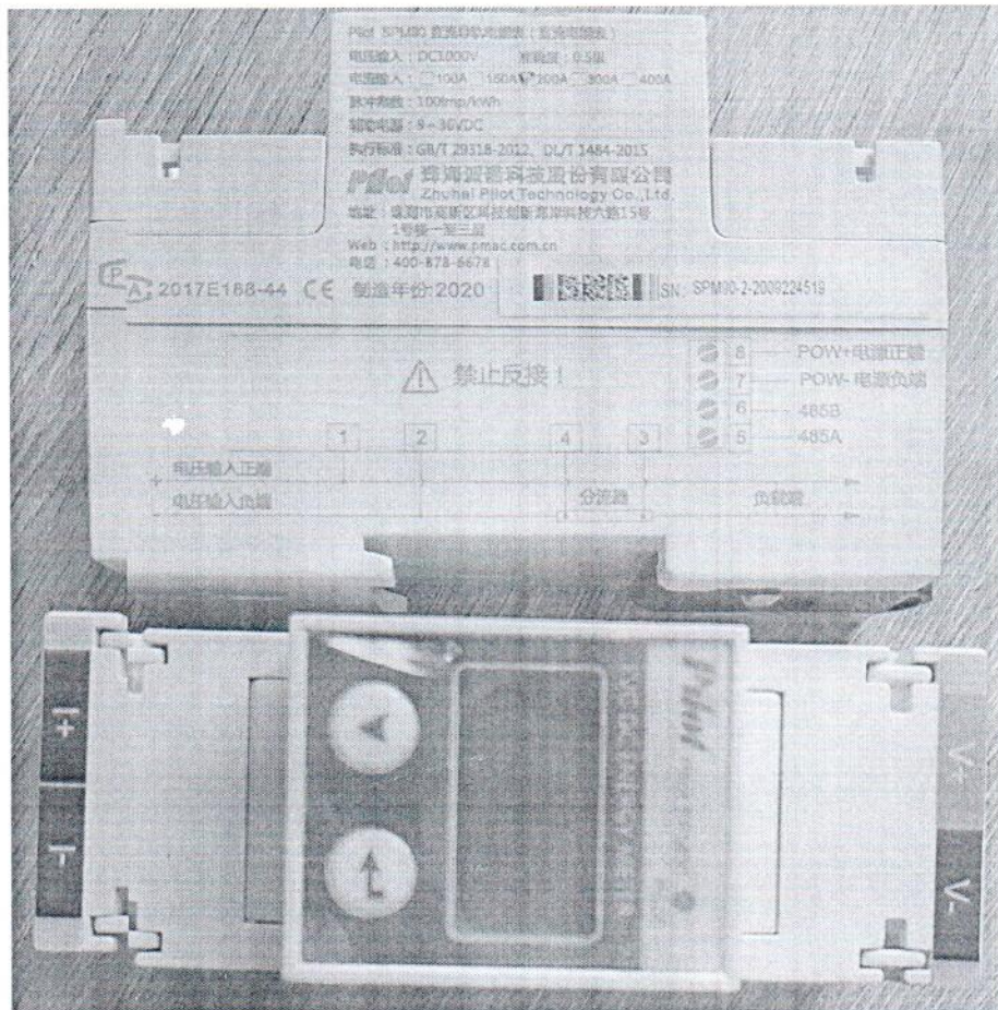
Рисунок 1.1 – Внешний вид счетчика SPM90 зав. № SPM90-2-2009224519
