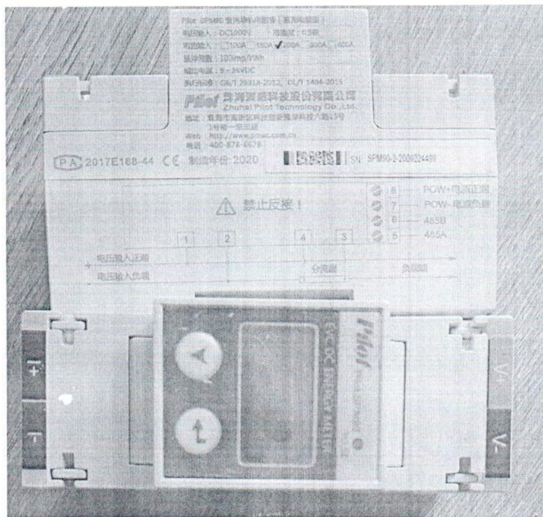
Рисунок 1.1 – Внешний вид счетчика SPM90 зав. № SPM90-2-2009224499
