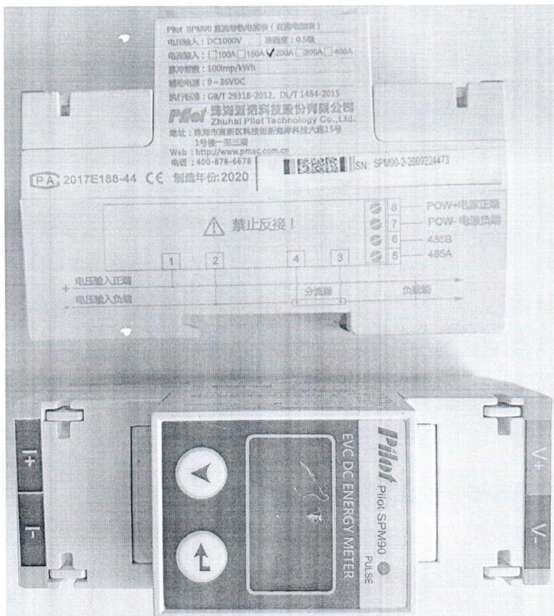
Рисунок 1.1 – Внешний вид счетчика SPM90 зав. № SPM90-2-2009224473
